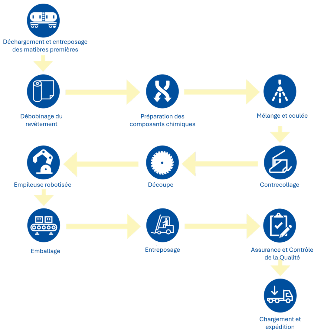
Figure 4. Fabrication des panneaux isolants en polyiso
