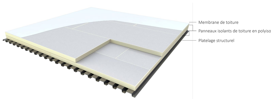
Figure 3. Installation type, avec panneaux de toiture posés directement sur le platelage
