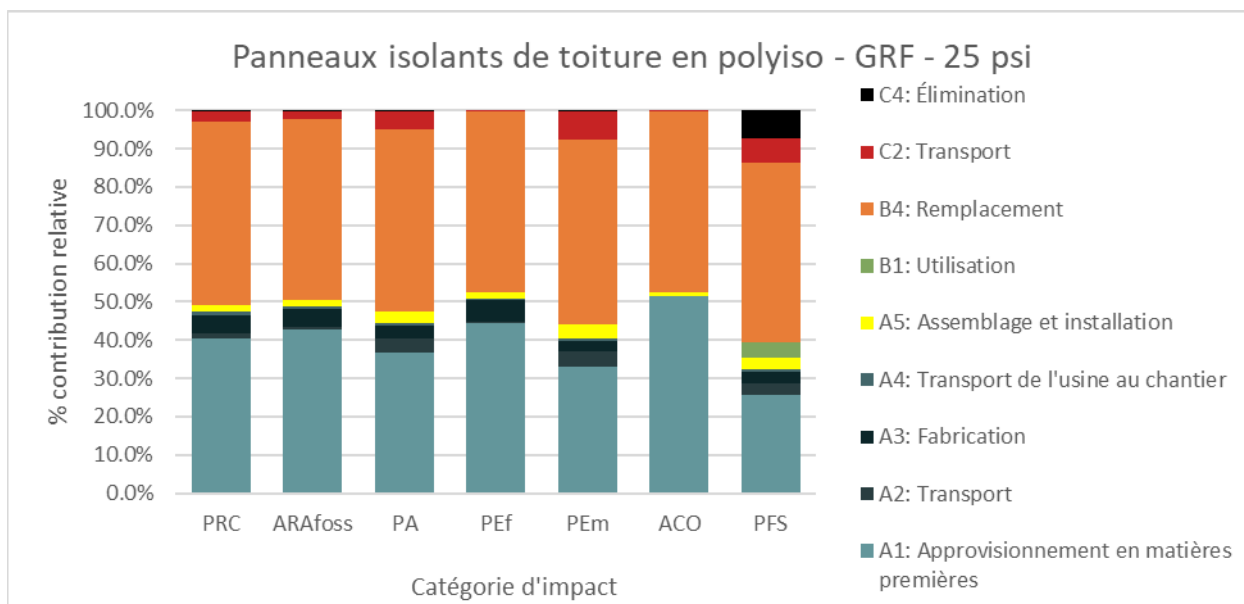
Figure 9. Contribution des différents modules du cycle de vie aux impacts environnementaux potentiels de 1 m² de panneau de toiture isolant en polyiso installé (type GRF 25 psi), pendant 75 ans
