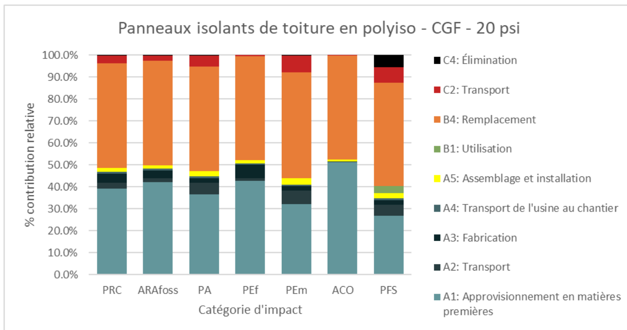
Figure 6. Contribution des différents modules du cycle de vie aux impacts environnementaux potentiels de 1 m 2 de panneau de toiture isolant en polyiso installé (type CGF 20 psi), pendant 75 ans
