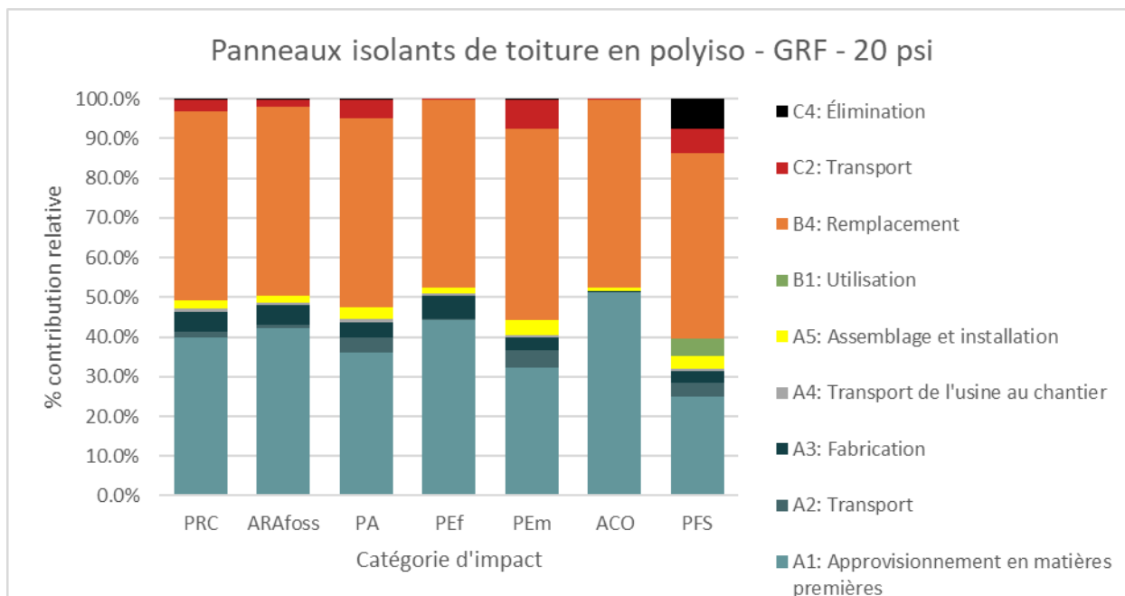
Figure 8. Contribution des différents modules du cycle de vie aux impacts environnementaux potentiels de 1 m² de panneau de toiture isolant en polyiso installé (type GRF 20 psi), pendant 75 ans
