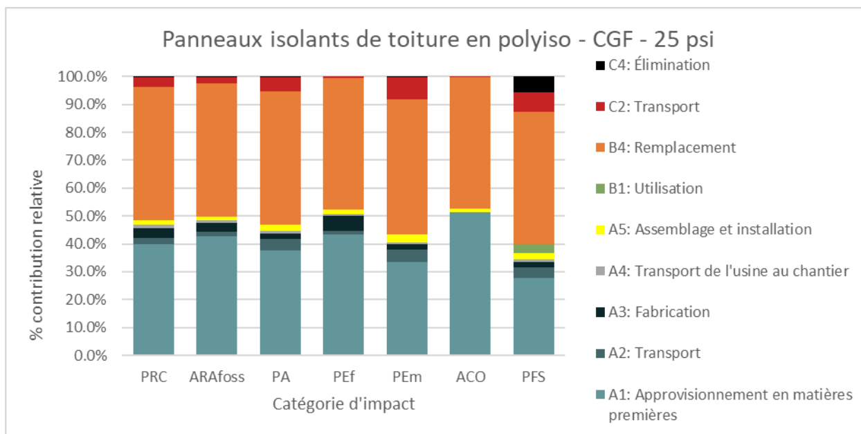
Figure 7. Contribution des différents modules du cycle de vie aux impacts environnementaux potentiels de 1 m 2 de panneau de toiture isolant en polyiso installé (type CGF 25 psi), pendant 75 ans
